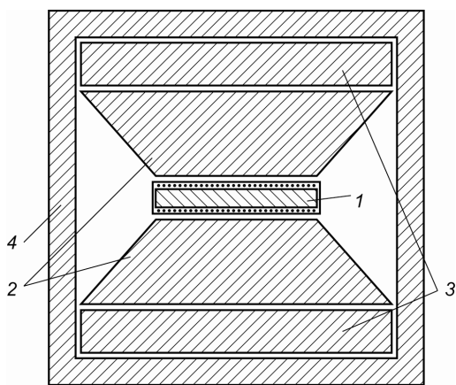
Рис. 1. Конструкция геликонового вентиля. 1 – геликоновый резонатор с катушками связи, 2 – полюсные наконечники, 3 – постоянные магниты, 4 – корпус вентиля.
