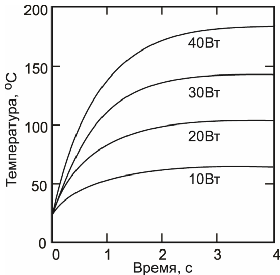
Рис.2. Расчетная зависимость температуры геликонового резонатора от времени после скачкообразного рассогласования нагрузки при различных мощностях передатчика.
