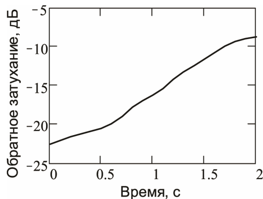
Рис.5. Зависимость обратного затухания геликонового вентиля от времени после скачкообразного рассогласования нагрузки.
