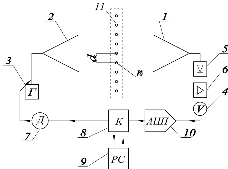
Рис. 4. Структурна схема вимірювального стенду
