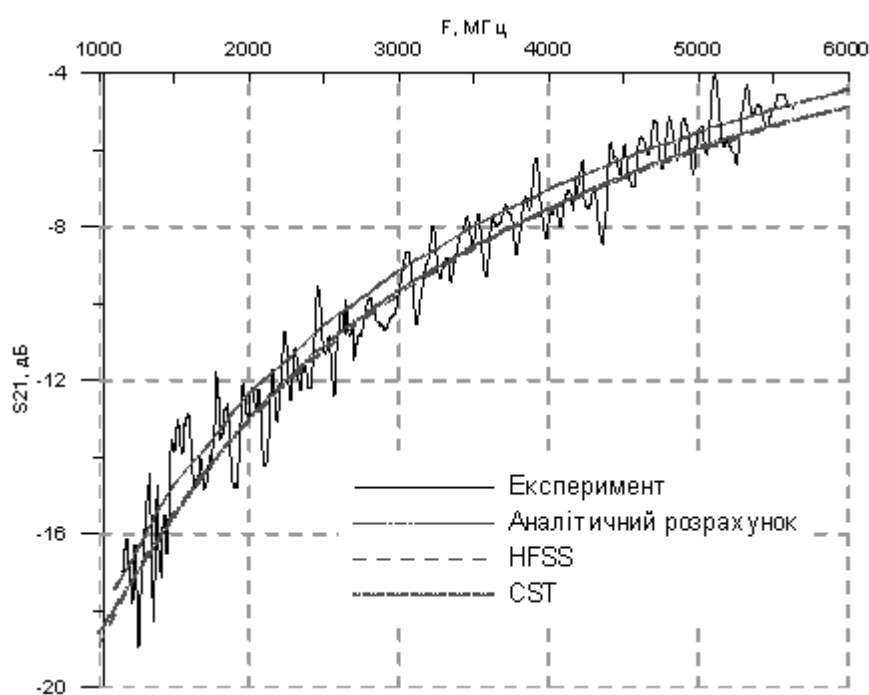
Рис. 5. Експериментальна та теоретичні залежності коефіцієнта проходження електромагнітної хвилі через осепаралельну сітку
