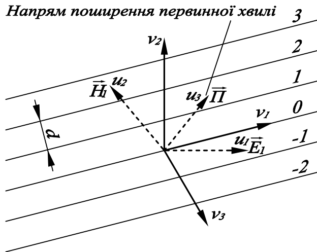
Рис.1. Системи координат та їх прив'язка до сітки і фронту хвилі
